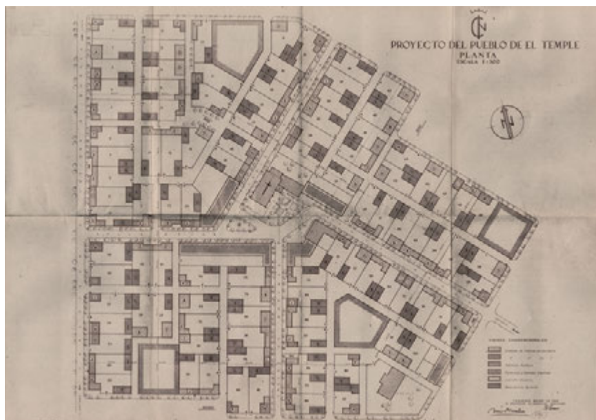
Planta general de El Temple. Proyecto de José Borobio, 1947. (AHPZ, «Pueblo de El Temple. Proyecto de cien viviendas con sus dependencias agrícolas para colonos. Tomo II. Planos»)
