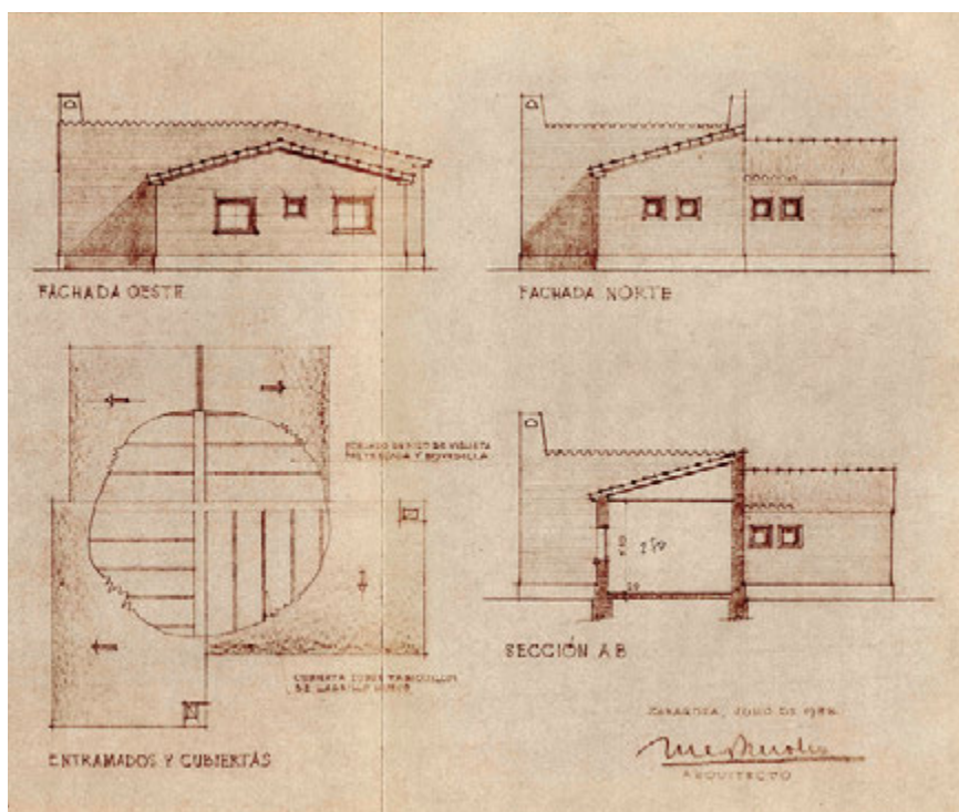
Perspectiva, fachadas, plantas y secciones del hogar rural para la Sección Femenina. José Borobio, 1958. (AHPZ, «Pueblo de El Temple. Proyecto de hogar rural de la Sección Femenina»)
