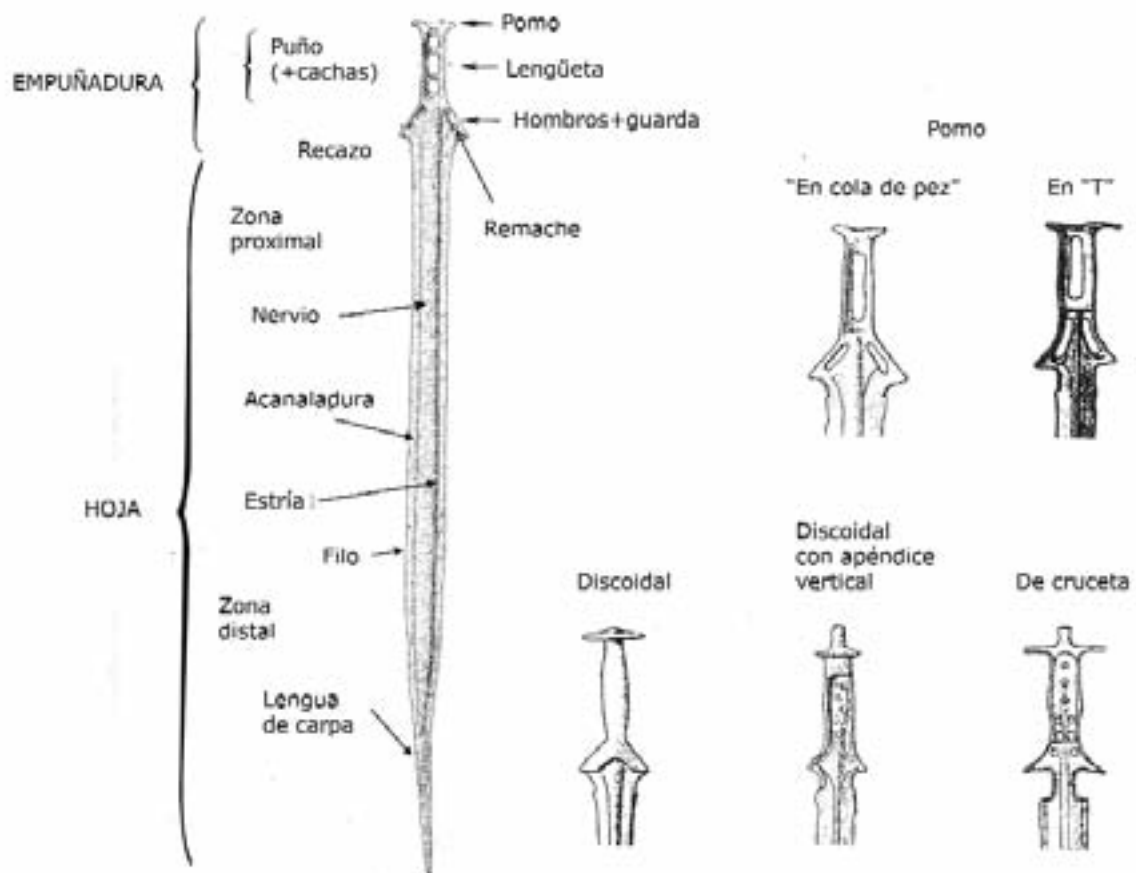
Partes de la espada de lengüeta (modificado sobre original de Farnié y Quesada, 2005).
